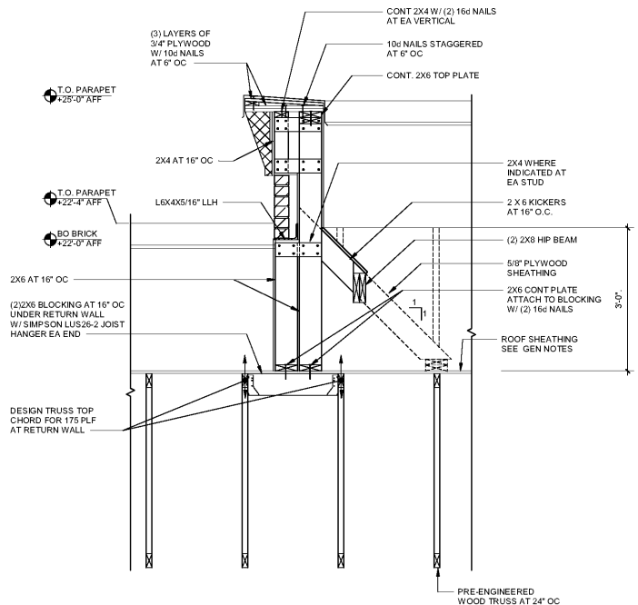
SECTION 214 SCALE: 3/4" = 1'-0"
